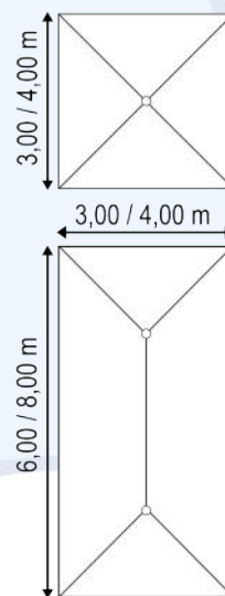
Draufsicht (nur obige Beispiele)
