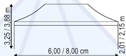
Seitenansicht (am Bsp. der 6 & 8 m Zelte)
